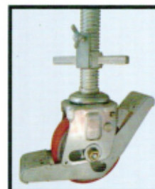
Particolare ruota AR-RL
